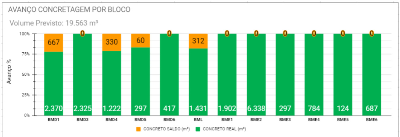
Figura 15 – Avanço concretagem por bloco (Vol. Real. Acum.: 18.192 m 3 )
