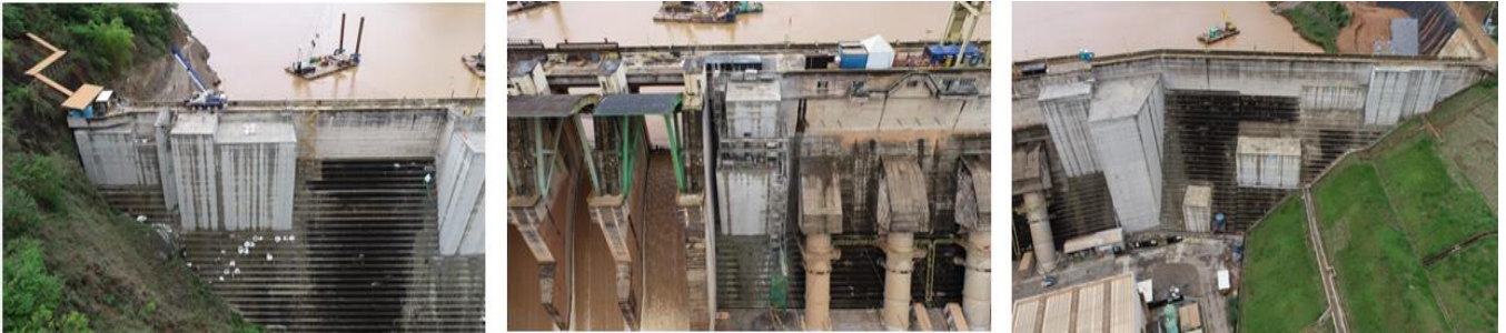
Figura 14 – Foto aérea blocos MD e ME
