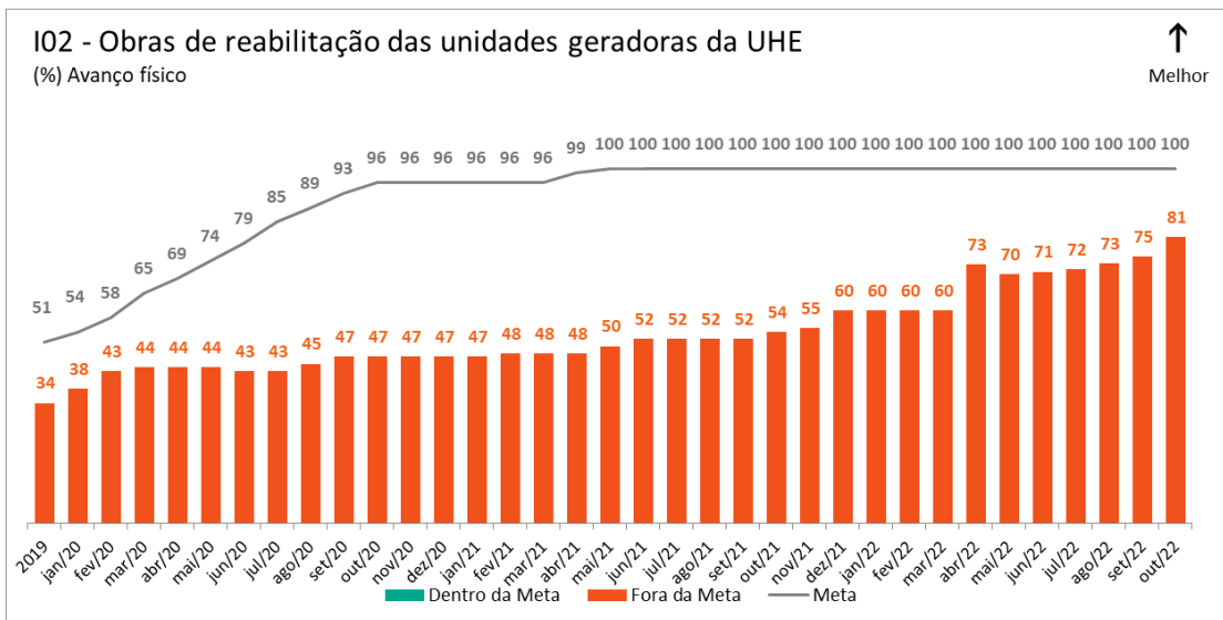
Gráfico 2 - Obras de reabilitação das unidades geradoras da UHE. Gráfico Acumulado.
